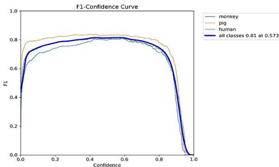
Fig. 6: F1 confidence curve.
