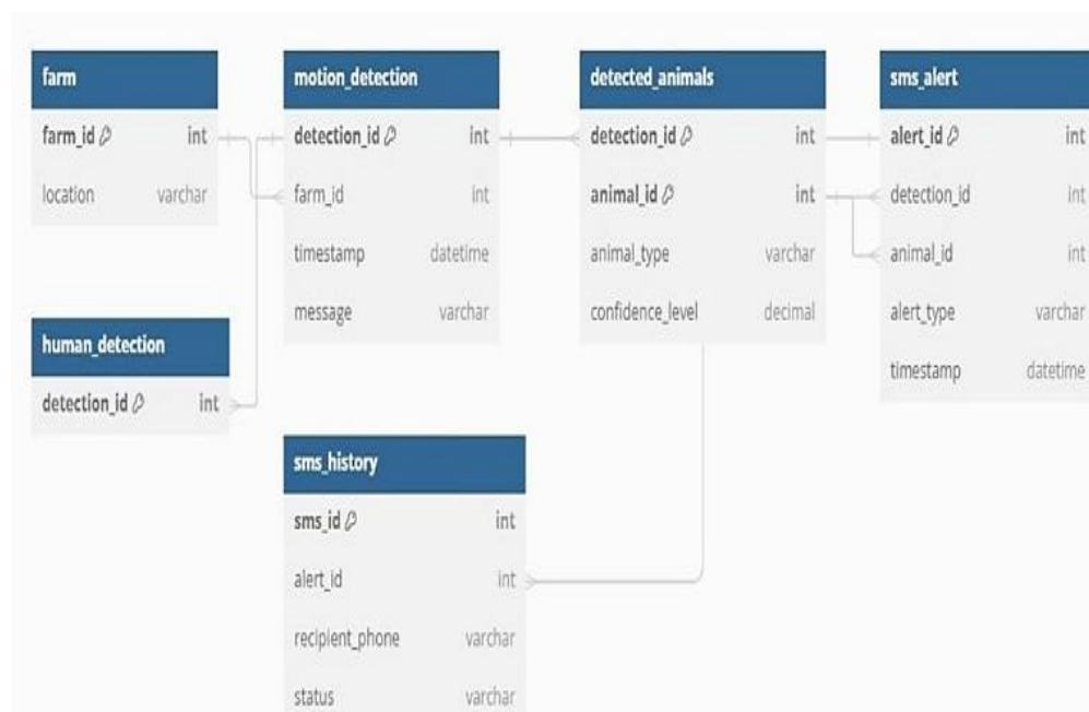
Fig. 3: Database diagram.
