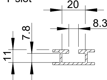
T-Slot/ T-slot
